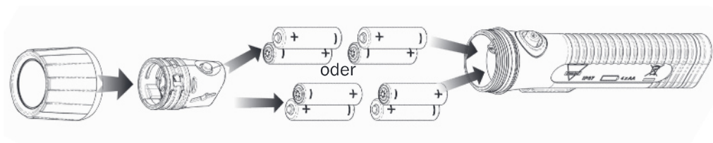
Bild 5: Explosionszeichnung HL 10 EX Typ 4920... mit Batterien
