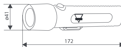
Bild 4: Abmessungen HL 10 EX 4920...
